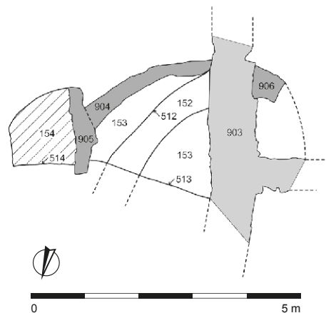
Obr. 63. Litovel. Zjednodušený půdorys pece a předpecní jámy po začištění povrchu. Kresba J. Novák, J. Grégr.
