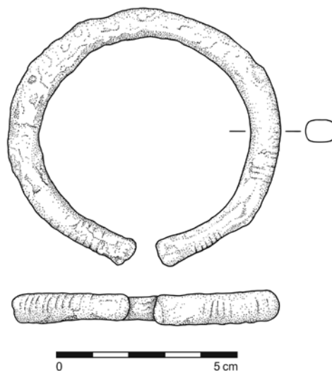
Obr. 11. Křenovice. Železný zdobený náramek. Kresba P. Holcová. Fig. 11. Křenovice. Decorated iron bracelet. Drawing by P. Holcová.
