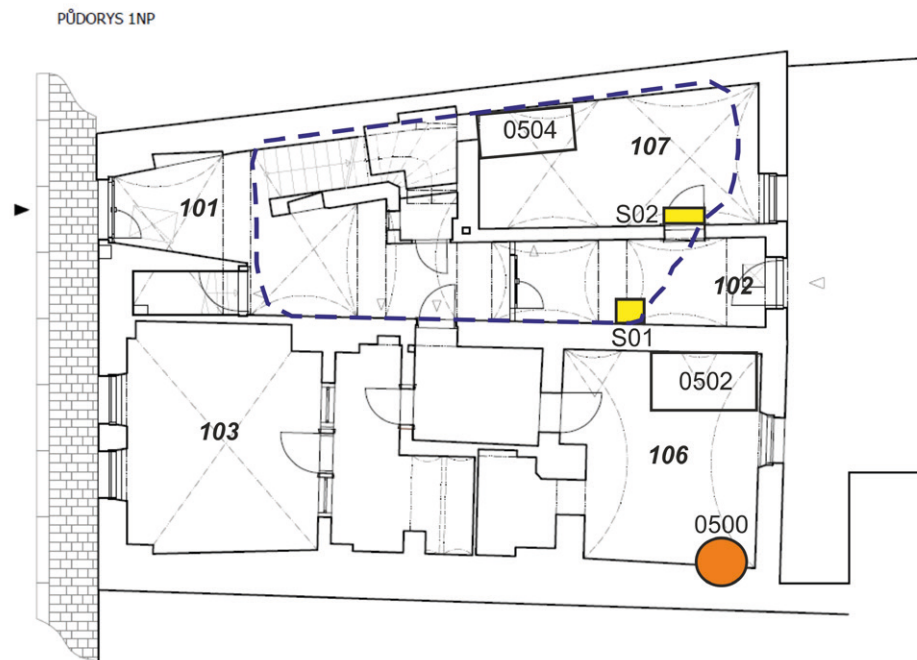
Obr. 50. Půdorys přízemí domu Havířská č. 6, Jihlava. 0500 jímka; přerušovanou čarou odhadovaný rozsah reliktu zahloubeného středověkého suterénu 0503; 0502 a 0504 novověké vápenné jámy (upraveno dle projektové dokumentace, autor P. Dvořák).
