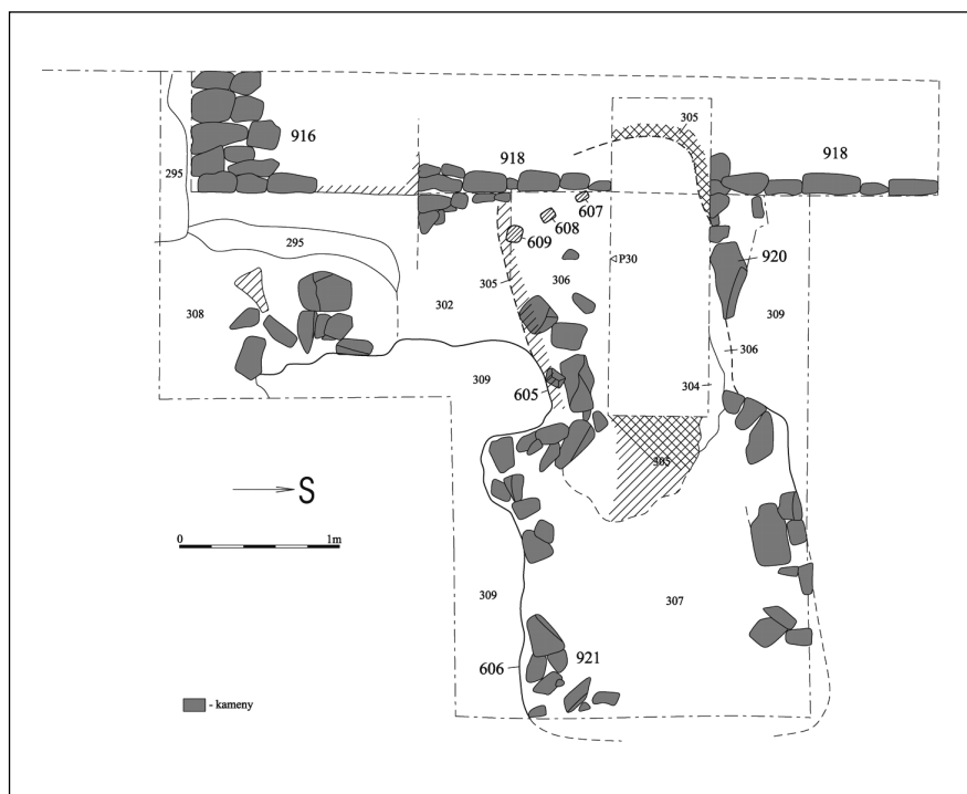
Obr. 96. Rajhrad – Městečko č. p. 52. Půdorys pece na vápno z pozdního středověku.
