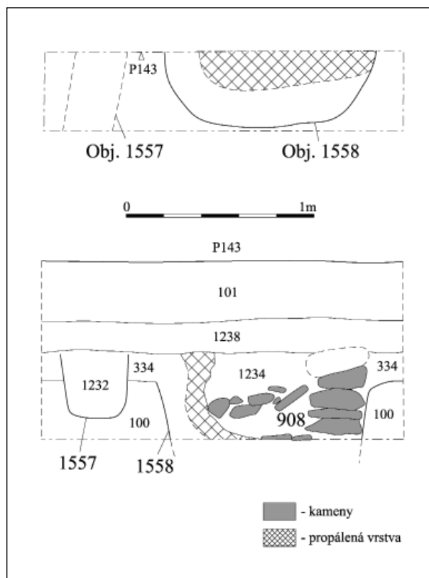
Obr. 43. Březí. Zaniklá středověká osada Bratelsbrunn. Řez peci.
