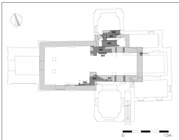
Obr. 85: Kunštát, Náměstí Krále Jiřího. Vyznačení odkrytých zděných konstrukcí. Abb. 85: Kunštát, König-Georg-Platz. Bezeichnung der dokumentierten Mauern.
