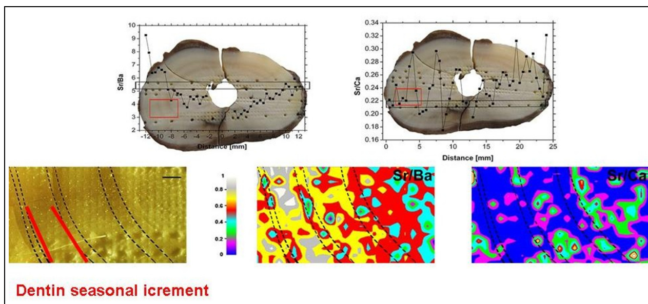
Fig. 6: The Sr/Ca and Sr/Ba ratios derived from LIBS line scan and LA-ICP-MS mapping. With dotted lines the different regions on the teeth cross section are shown. The bar has a length of 500 \mu m. Obr. 6: Poměr Sr/Ca a Sr/Ba odvozený z line scanu měřeného pomocí metod LIBS a LA-ICP-MS mapování. Tečkovanou čarou jsou vyznačeny oblasti zimních a letních přírůstků dentinu. Škála má délku 500 \mu m. Dental seasonal increment = sezónní přírůstky dentinu.
