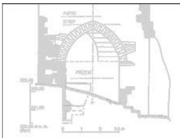
Obr. 90. Olomouc, Mlčochova, Dobrovského ulice. Detail soutisku profilu P 1 s nárysem sz stěny brány Všech svatých (podle Kšír 1967, 54). Abb. 90. Olmütz, Mlčochova, Dobrovského Str. Detail des Profils P 1 mit der nordwestlich orientierten Mauer beim Allerheiligen-Stadtor (nach Kšír 1967, 54).
