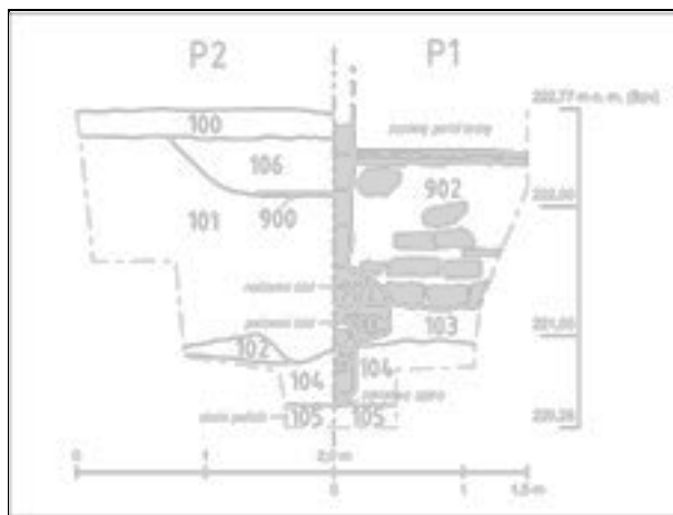
Obr. 89. Olomouc, Mlčochova, Dobrovského ulice. Sonda S 1/10 u městské brány Všech svatých, profily P 1–2. Abb. 89. Olmütz, Mlčochova, Dobrovského Str. Sondage S 1/10 beim Stadtor der Allerheiligen, Profile P 1–2.
