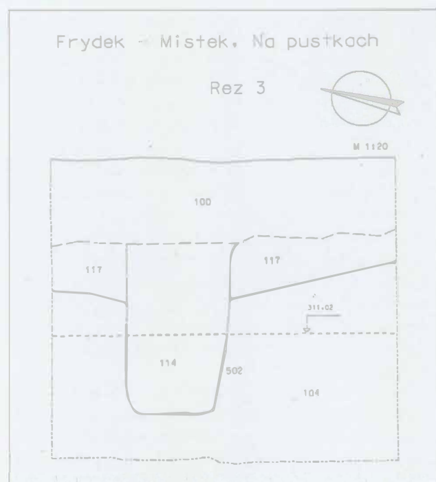
Obr. 54: Frýdek-Místek, ulice Na Půstkách a Na Blatnici. Řez odpadní jámou z 18. století. Fig. 54: Frýdek-Místek, Na Půstkách and Na Blatnici Streets. Section of a garbage pit from 18th century.
