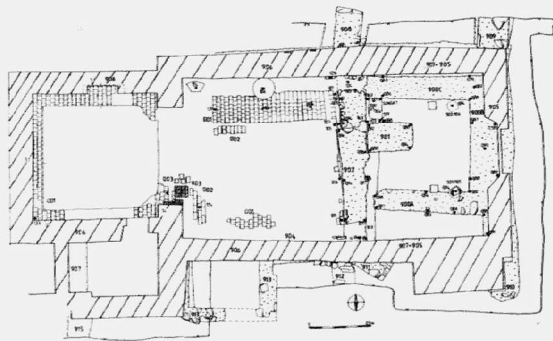
Obr. 141. Miroslavské Knínice – kostel sv. Mikuláše. Celkový půdorys kostela s odkrytými zdivy starších stavebních fází.
