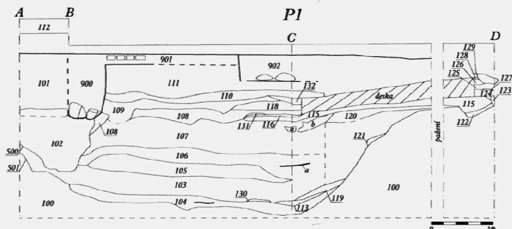
Obr. 142. Modřice, Havlíčkova ulice, č. p. 187. Profil P1 se středověkým zahloubeným objektem č. 501. Modřice, Havlíčkova Str., Kon. N. 187. Schnitt P1 mit der mittelalterlichen Grube N. 501.
