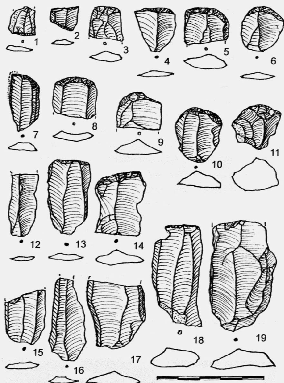
Obr. 18. Tučapy. Výběr Kamenné industrie. Tučapy. Steinindustrie (Auswahl).
