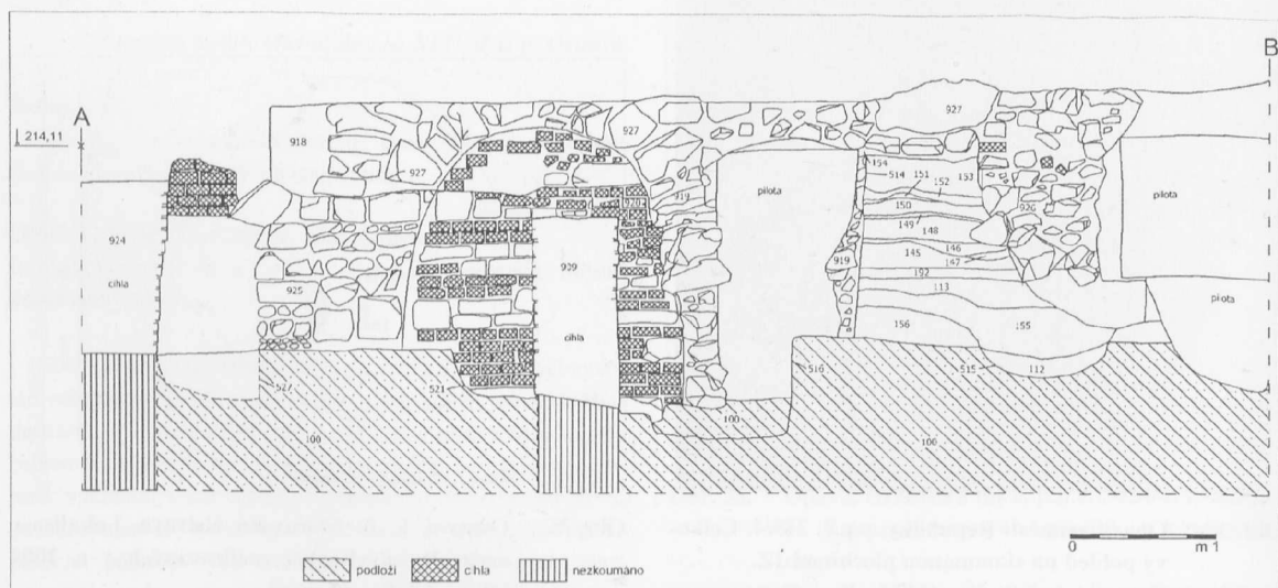
Obr. 36. Ostrava, Masarykovo nám. 32. Profil A-B na SZ stěně stavební jámy. Ostrava, Masarykovo Platz. 32. Suchschnitt A-B.
