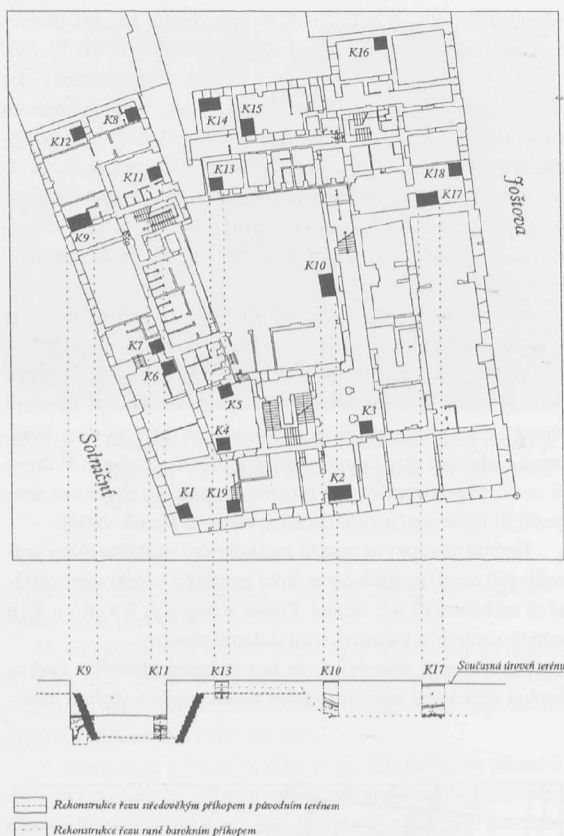
Obr. 50. Moravské náměstí 6 (A013/2004). Rozmístění sond. Dole rekonstruované řezy středověkého a raně barokního příkopu. Moravské náměstí 6 (A013/2004). Verteilung der Suchschnitte. Unten rekonstruierte Profile des mittelalterlichen und frühbarocken Grabens.
