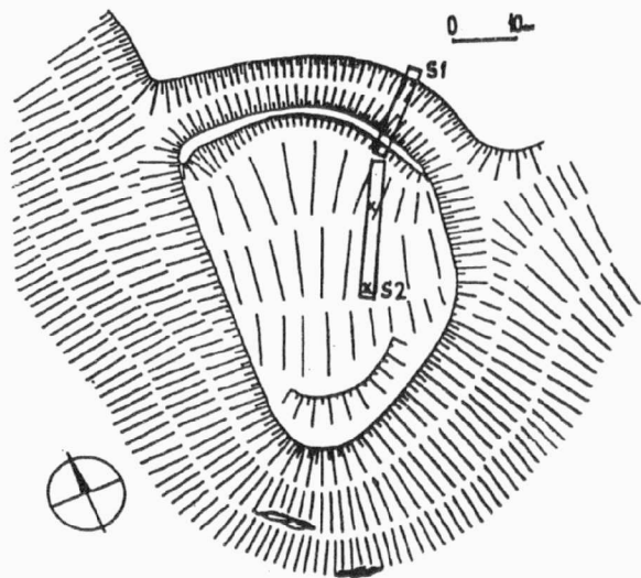
Obr. 7. Čekyně, Nad rozsypanou skálou. Terénní náčrt opevnění.
