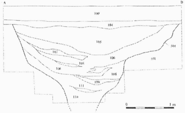
Obr. 2. Bedřichovice, Malá pole. Profil příkopu (spodní část nedokopána). Bedřichovice, Malá pole. Profil des Grabens (Forschung des unteren Teil ist nicht beendet).
