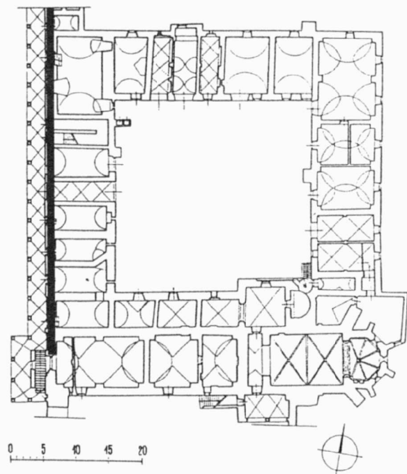
Obr. 29. Oslavany – klášter. Půdorys. Černě vyznačena dokumentovaná zeď. Oslavany – Kloster. Grundriß.
