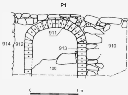
Obr. 1. Znojmo, minoritský klášter. Příčný řez vstupní šíjí novověké krypty. Znojmo, Minoritenkloster. Querschnitt durch den Eingangsteil der neuzeitlichen Krypte.
