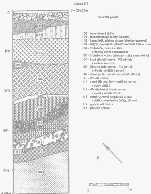
Obr. 37. Přerov – Horní náměstí, čp. 26 – stratigrafie sondy III. Přerov – Horní náměstí, Nr. 26 – Stratigraphie des Suchschnitts III.
