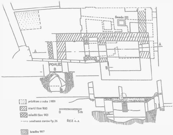
Obr. 36. Přerov – Horní náměstí, čp. 26 – půdorys domu s vyznačením sondy III. Přerov – Horní náměstí, Nr. 26 – Hausgrundriß mit Bezeichnung des Suchschnitts III.
