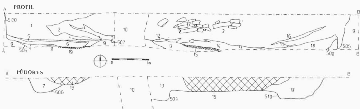
Obr. 13. Vyškov, nemocnice s poliklinikou. Profil a půdorys pece ze starší doby římské. Vyškov, Krankenhaus. Schnitt und Grundriß des Ofens der älteren römischen Kaiserzeit.
