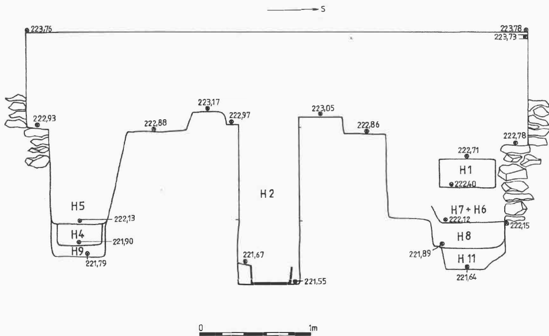
Obr. 1: Prostějov, augustiniánský klášter. Schematický profil presbytáře kaple.
