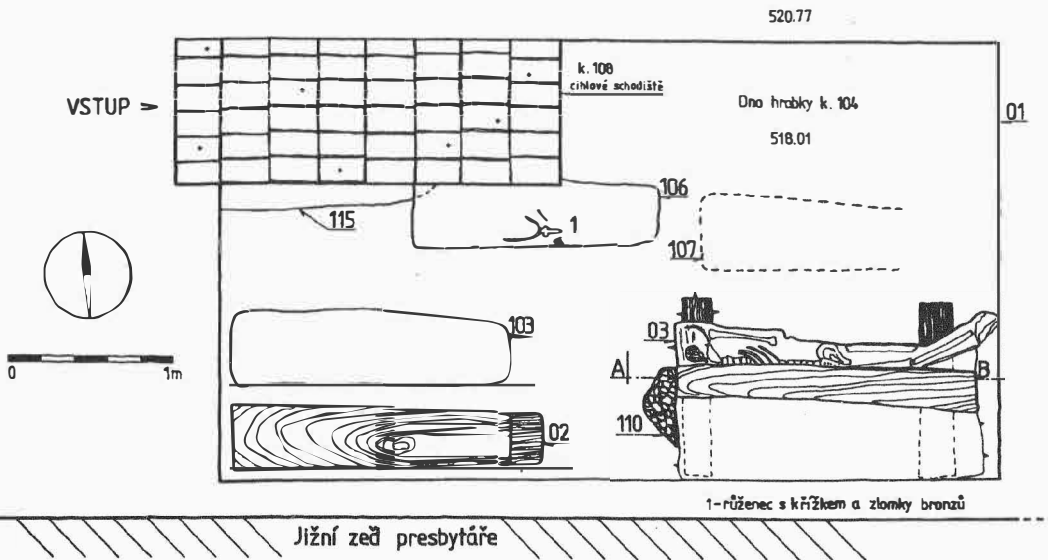
Obr. 1. Jihlava, Křížová 4. Půdorys jižní hrobky v presbytáři kostela Povýšení Sv. Kříže. „Křížová“ Gasse Nr. 4. Der Grundriß der Südgruft im Chor der St. - Kreuz - Kirche.
